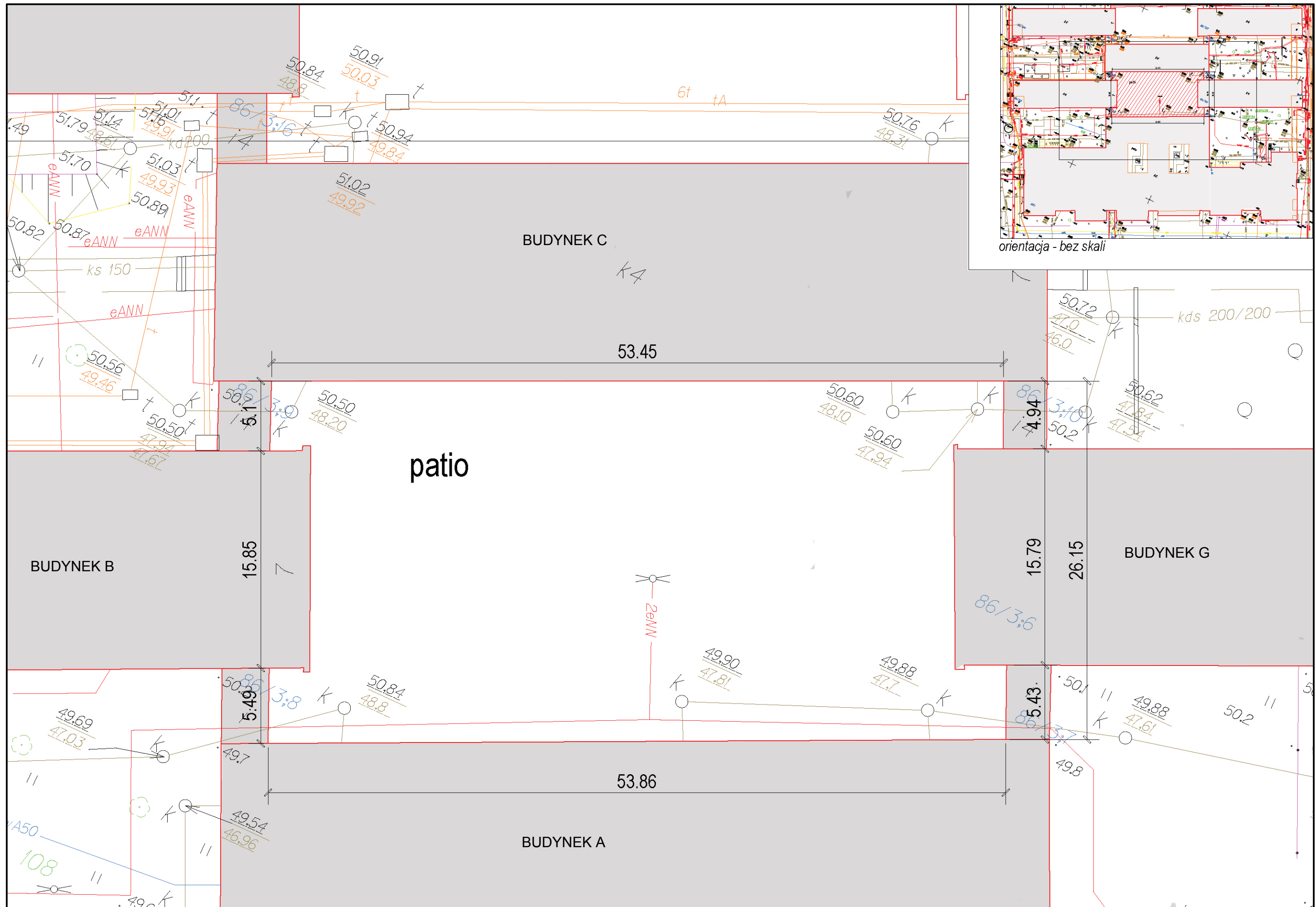
lokalizacja - skala 1:250
